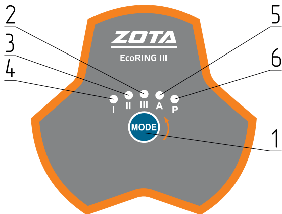
Рис.16 Органы управления.
