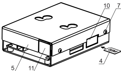
Рис.3 Подключение модуля GSM/GPRS к плате управления БУ Zota Smart SE/МК-S/Solid
