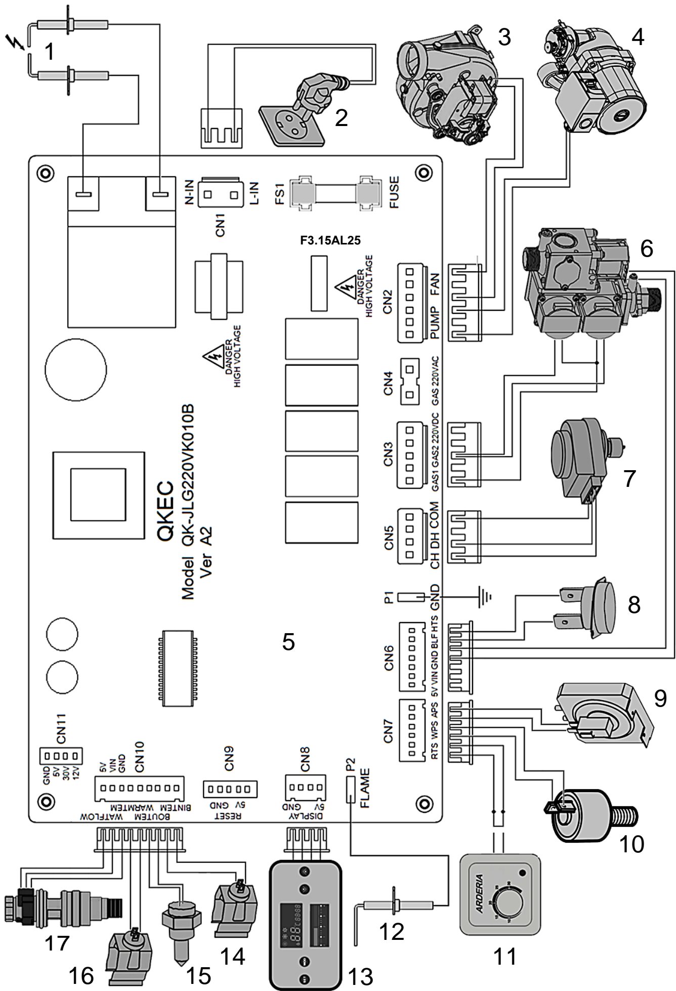
Рис. 42 Принципиальная электрическая схема котлов Arderia
